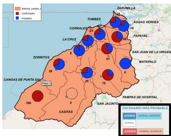
Gráfico 9. Pronóstico climático de temperatura máxima y casos de dengue, Región de Tumbes, SE 01-09/2025
