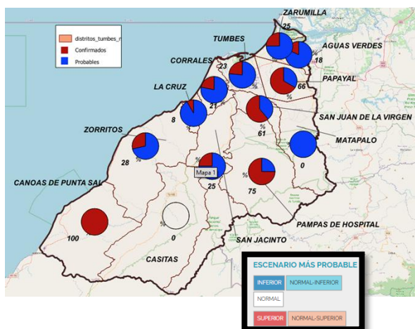
Gráfico 10. Pronóstico climático de temperatura mínima y casos de dengue, Región de Tumbes, SE 01-09/2025
