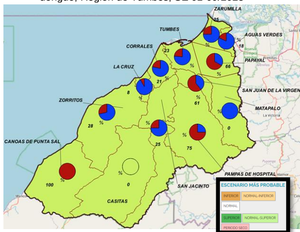
Gráfico 8. Pronóstico climático de precipitaciones y casos de dengue, Región de Tumbes, SE 01-09/2025
